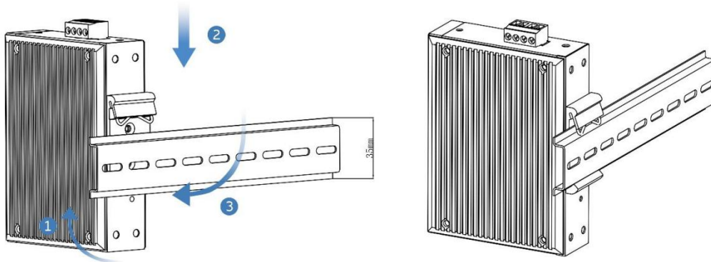
安装示意图
