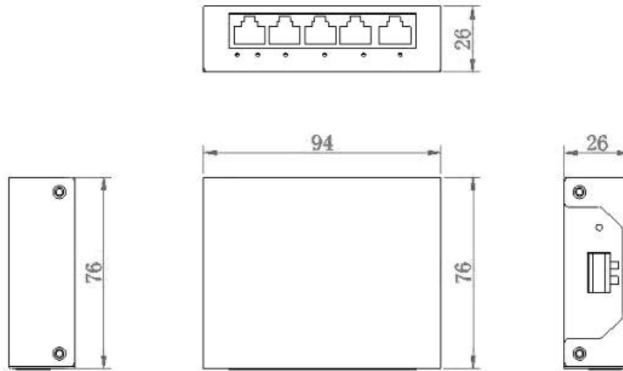
CMS-S05M 外形尺寸图
